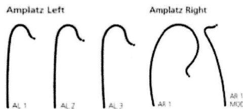
Fig. 1: Catéter diagnóstico coronario tipo amplatz (no incluye diseño)
