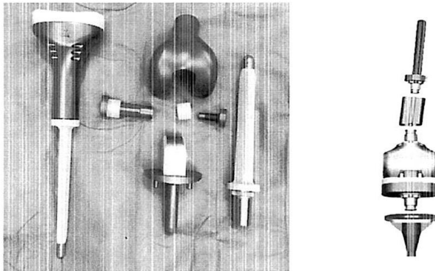
Fig. 1.: Prótesis tumoral de Fémur Distal (no incluye diseño)
